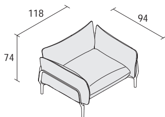
VINA V01
